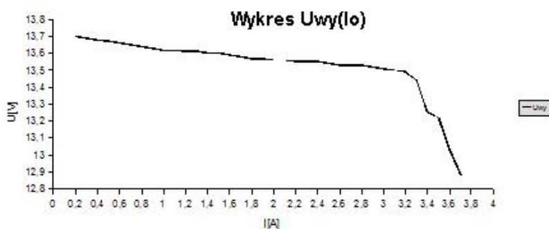
Rys. 4. Charakterystyka prądowo-napięciowa zasilacza.
