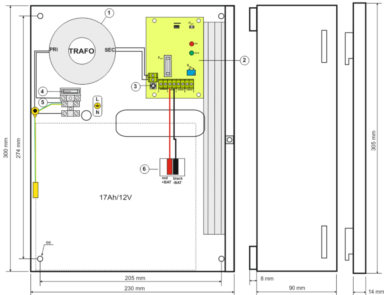
Rys.3. Widok zasilacza.
