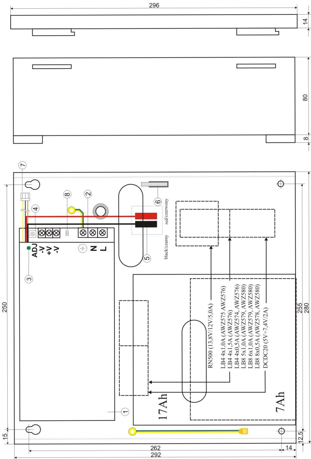
Rys.2. Widok zasilacza.
