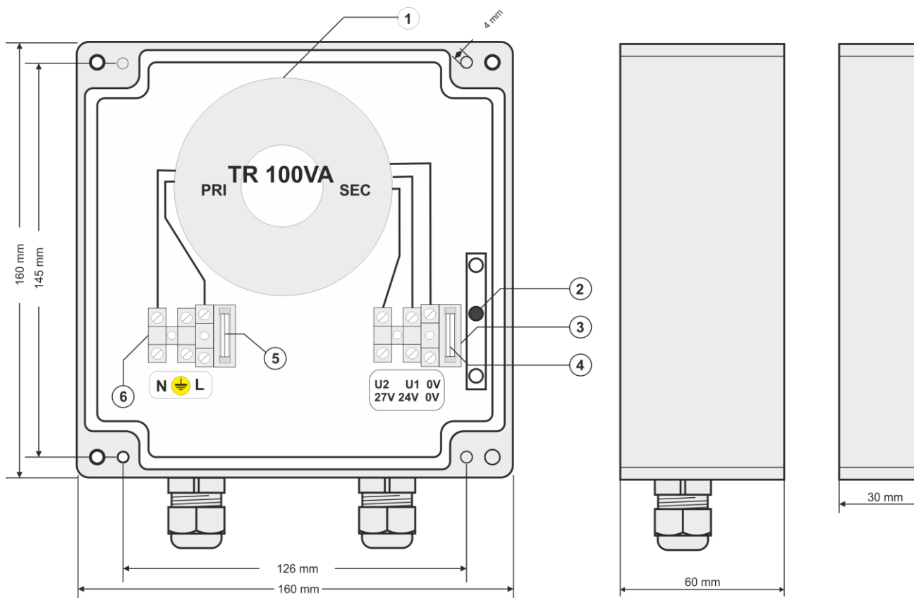
Rys.2. Widok zasilacza.
